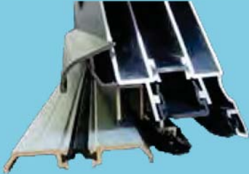
Seuil alu 10mm, à rupture de pont thermique
