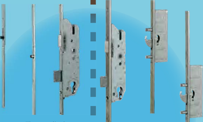
855 GL T11 verrouillage par relevage de béquille Gâche filante
